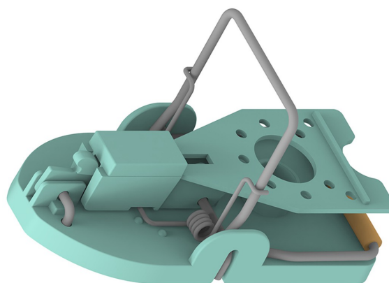
立体图
